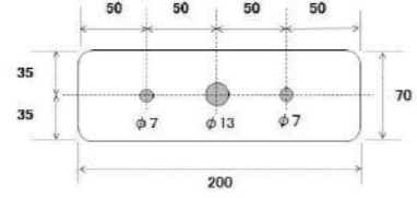
ランプ裏面 (取付け穴加工)
